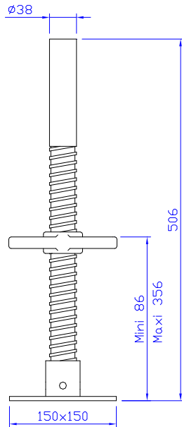
Socle réglable
