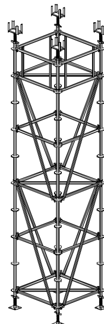
Tour d'étalement
